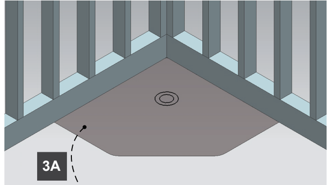
Floor leveling compound or mortar Ciment égalisateur ou mortier
